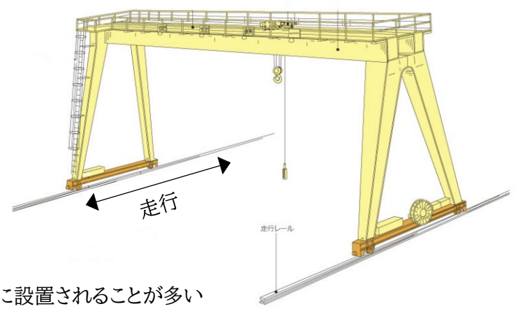
C : 橋形クレーン
